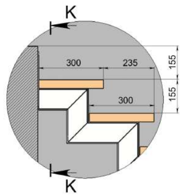
Д (1 : 6)
