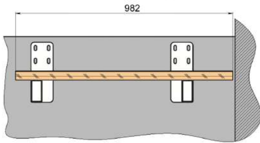
К-К (1 : 6)
