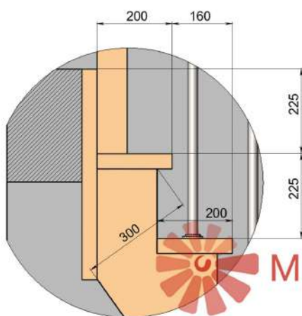
А (1 : 5)
