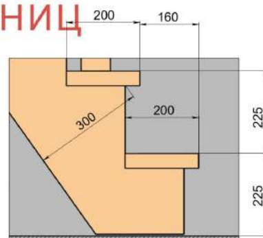
Б (1 : 5)
