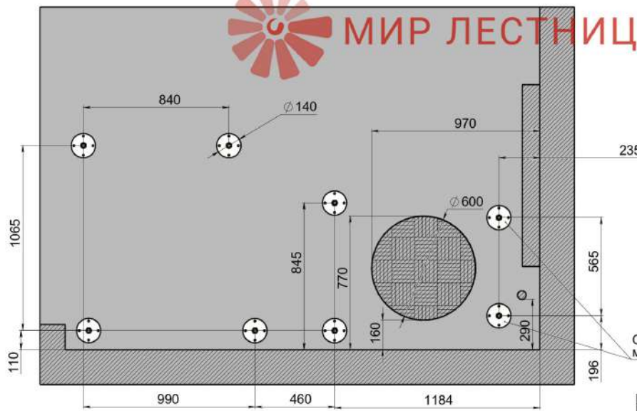
В-В (1 : 11)
