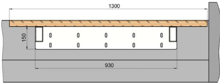
В-В (1 : 11)
