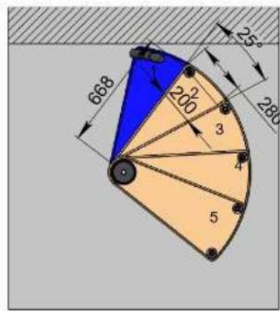
Б-Б (1 : 21)
