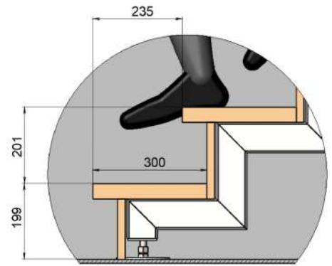
Б (1 : 5)
