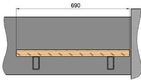
В-В (1 : 10)
