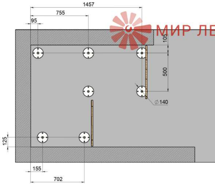
В-В (1 : 10)
