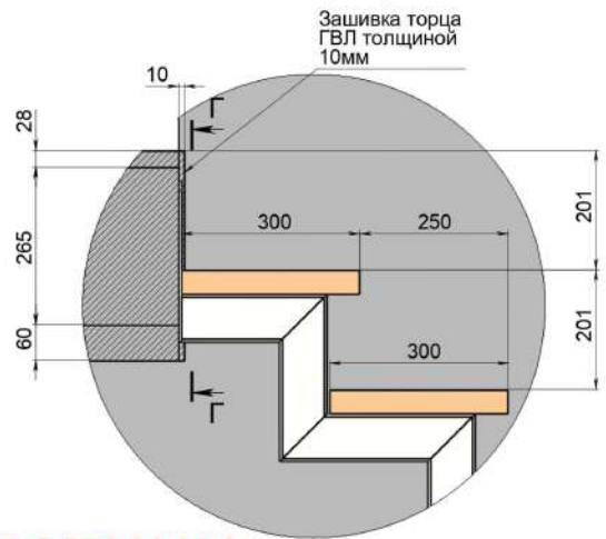
Б (1 : 5)
