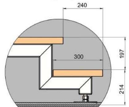
Б (1 : 5)
