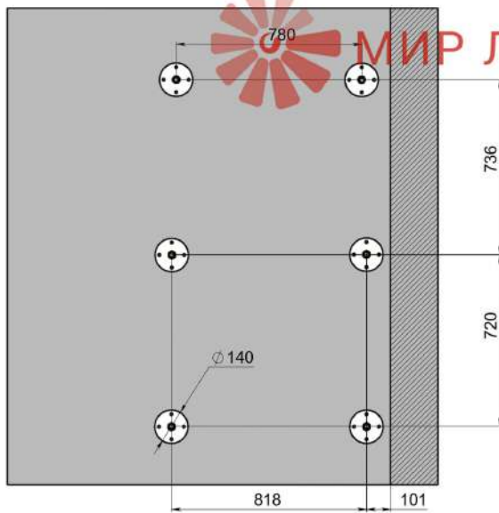
В-В (1 : 10)
