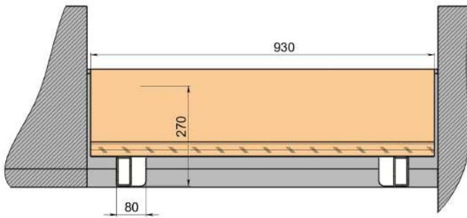
Е-Е (1 : 5)
