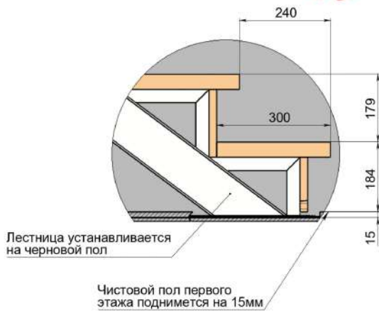
Г (1 : 5)
